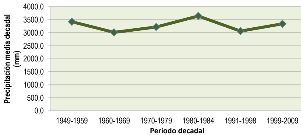
Gráfico No. 5 Tendencias anuales de precipitación en la estación M027 (aeropuerto)
